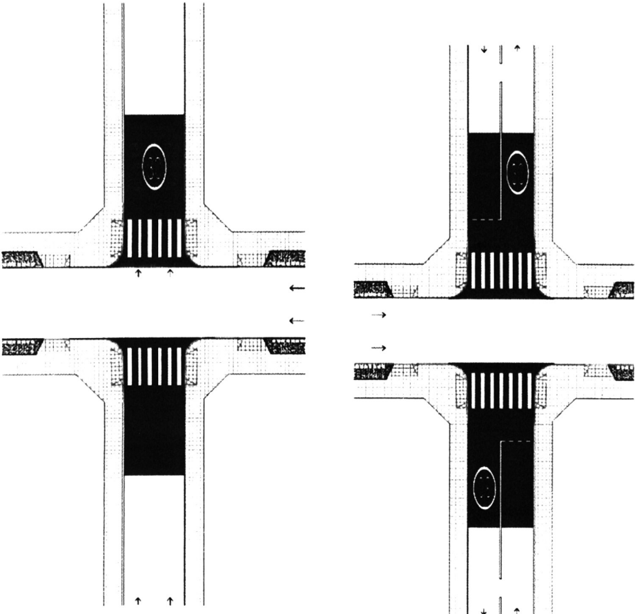
Demarcación calle un sentido; cruce con Paso Cebra
