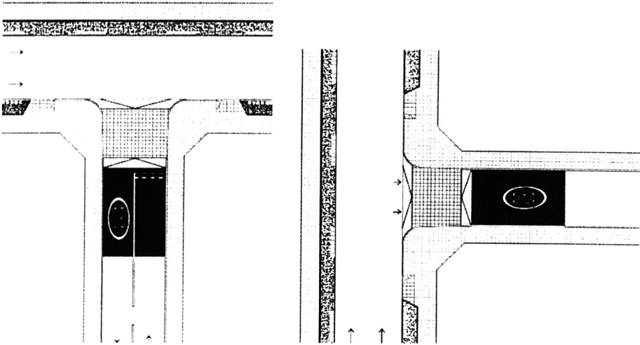
Demarcación con vereda continua, calle 2 sentidos.
