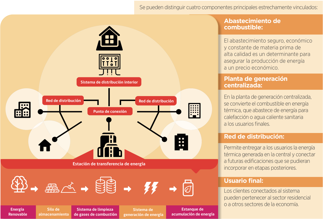
Figura 1-2: Vista general de la cadena de producción de un sistema de Energía Distrital
