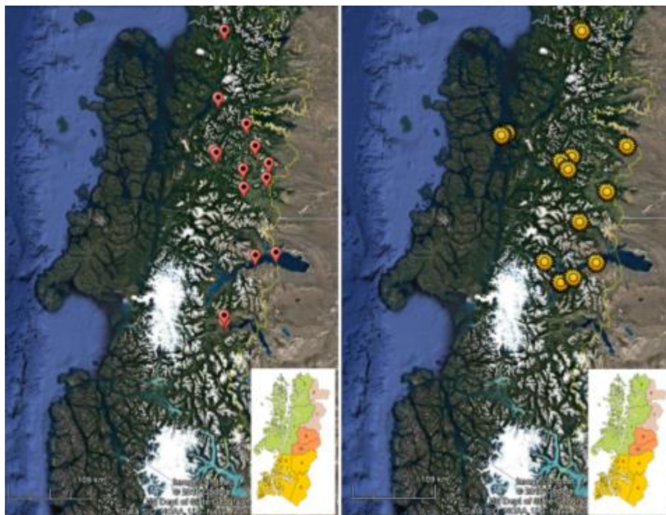
Ilustración 25: Proyectos de Electrificación Rural: Extensión de Red (izquierda) y Autogeneración (derecha). Fuente: Seremi de Energía, con datos a diciembre de 2016.
