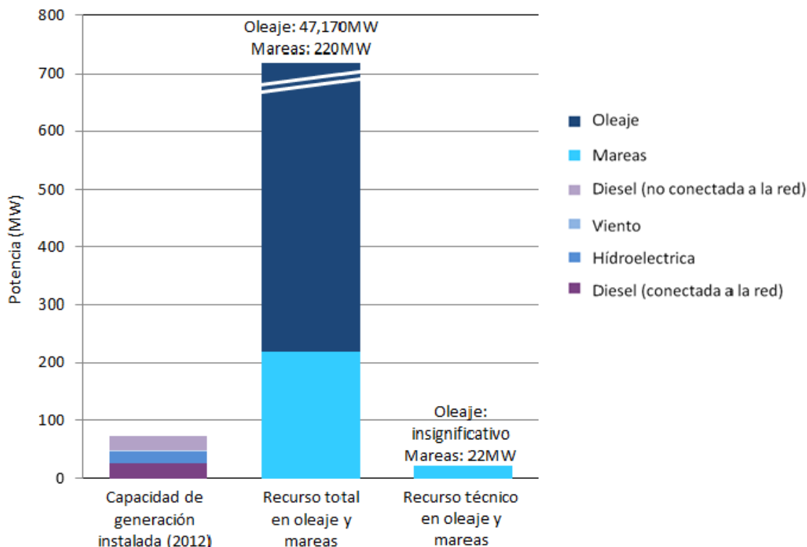
Ilustración 31: Capacidad instalada de generación comparada con los recursos de energía marina bruto y técnico para la Región de Aysén. Fuente: Aquatera (2014).
