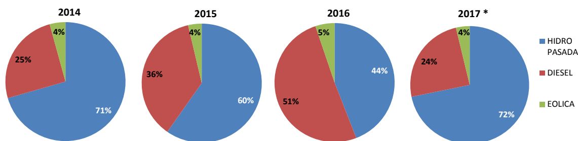
Ilustración 22: Generación bruta de los sistemas medianos de Aysén, 2014-2017. (*) Datos 2017 a mayo. Fuente: CNE.
