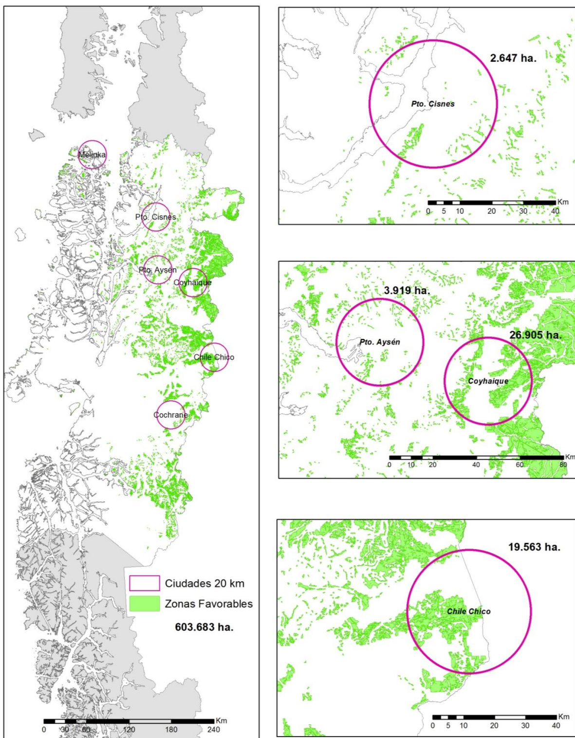
Ilustración 26: Zonas con alto potencial eólico cercano a centros de consumo. Fuente: Ministerio de Energía.
