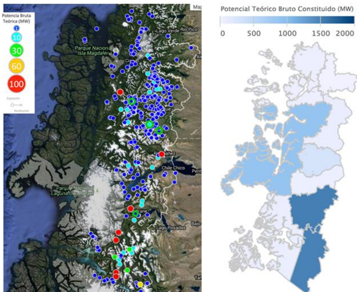
Ilustración 28: Izq. Distribución de los derechos de aprovechamiento de aguas no consuntivos (DAANC) de la Región de Aysén. Der. Potencial teórico bruto de las comunas de Aysén, determinado en base a los DAANC ya otorgados en la región. Fuente: U. de Chile (2015).
