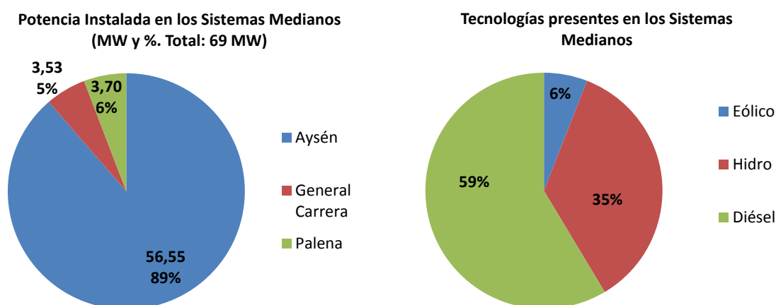
Ilustración 21: Sistemas Medianos de Aysén: Potencia Instalada (izq.) y Tecnologías (der.). Fuente: Seremi de Energía de Aysén.
